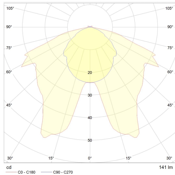
Lichtverteilungskurve
