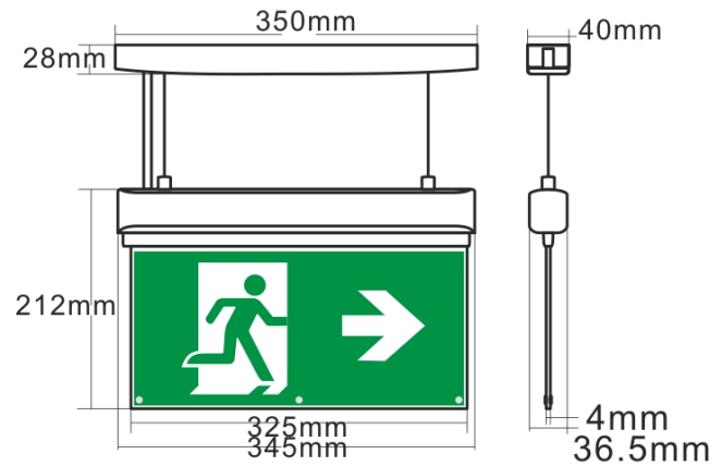
Maßskizze
