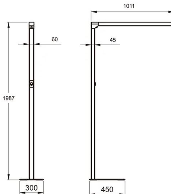
Maßskizze
